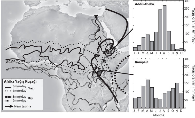
ŞEKİL 15. Nil'in yıllık taşkınlarının nem taşıma vektörleri. Blanchet, Contoux ve Leduc'tan (2015). Kalın çizgiler 6 mm/gün, noktalı çizgiler ise 3 mm/gün eşyağış eğrilerini göstermektedir.
