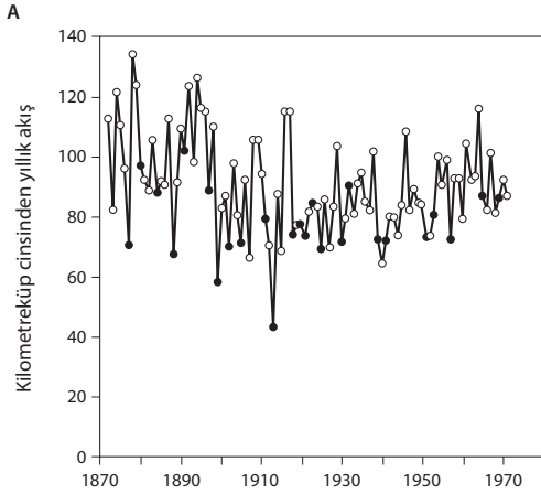
ŞEKİL 16. Üç farklı tarih aralığında Nil Nehri'nin yıllık dalgalanmaları; Edjga, Göl ve Katmai patlamalarından sonra kaydedilen düşük akışlara dikkat edin; sonuncusu muhtemelen 1902'de tamamlanan Aswan'daki alçak barajın aracılık ettiği bir durumdur. Umman ve diğ.den uyarlanmıştır. (2006)
